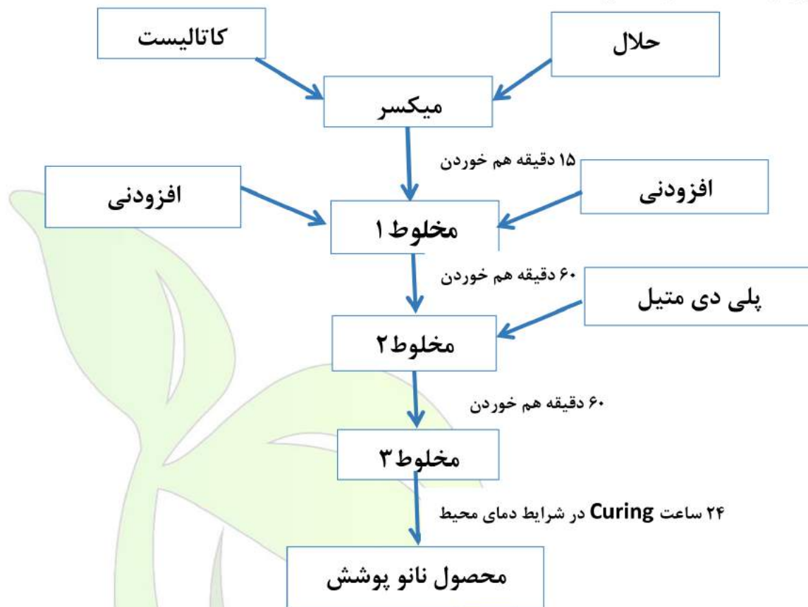
شکل ۲-۲ نمودار فرآیند عملیات تولید (OPC)
