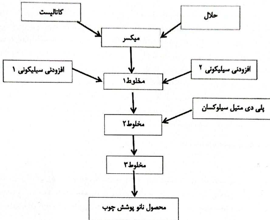
شکل ۴-۱ تصویر نمودار فرآیند تولید محصول شرکت نانو فراز سپاهان
