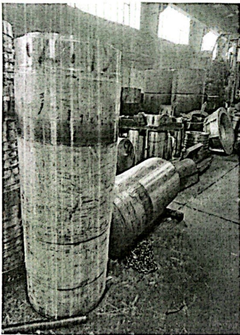
شکل ۴- تصاویری از عملیات فورج و ریخته گری
