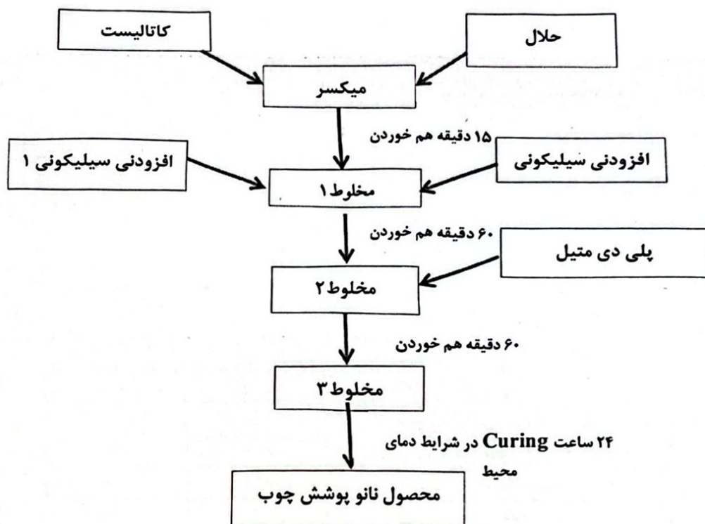
شکل ۴-۱ تصویر نمودار فرآیند تولید محصول شرکت نانو فراز سپاهان
